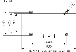
图5 (b) 底脚螺栓位置
